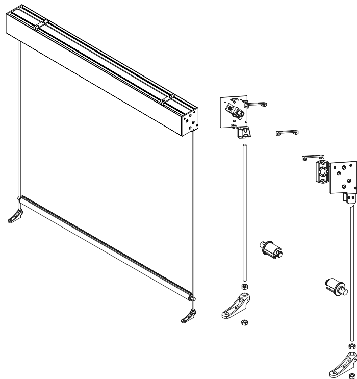
VENEZIA CASSONETTO QUADRO
